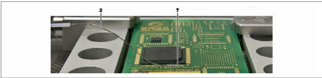
Abb. 35: Beispielabbildungen: Thermoelementhalter (oben) und Thermoelement platzieren (unten)
