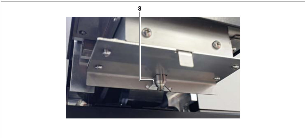
Abb. 33: Die ausgefahrene Pipette (3) in der Position zum Düsenwechsel. Das Bild zeigt die Pipette ohne aufgeschraubte Düse. Die Transportsicherung ist angebracht.
