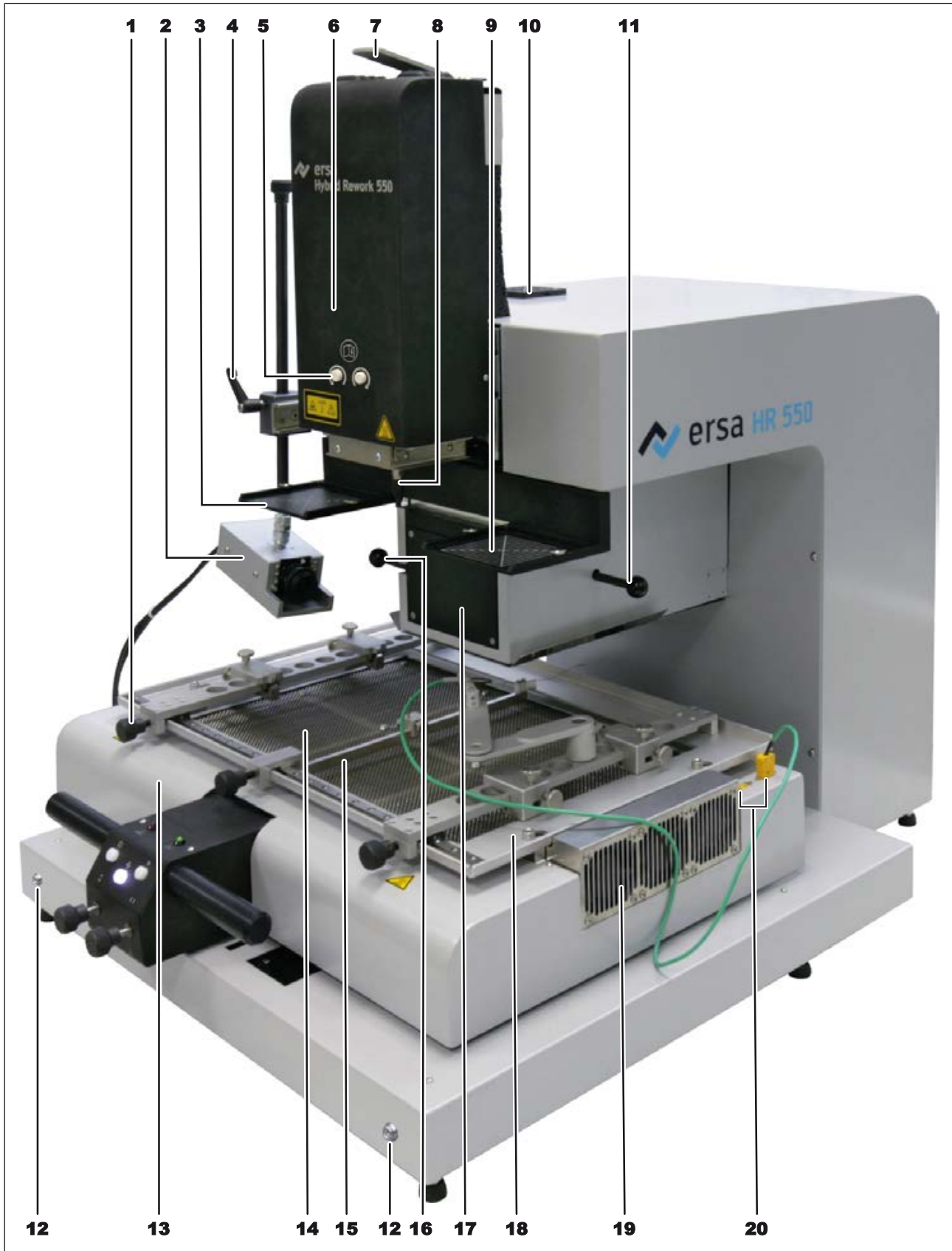
Abb. 24: Übersicht der Maschinenteile
