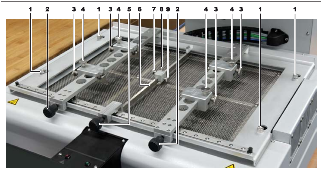
Abb. 30: Details des Leiterplattenrahmens
