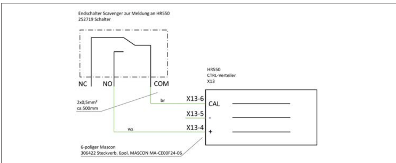
Abb. 18: Verdrahtungsplan
