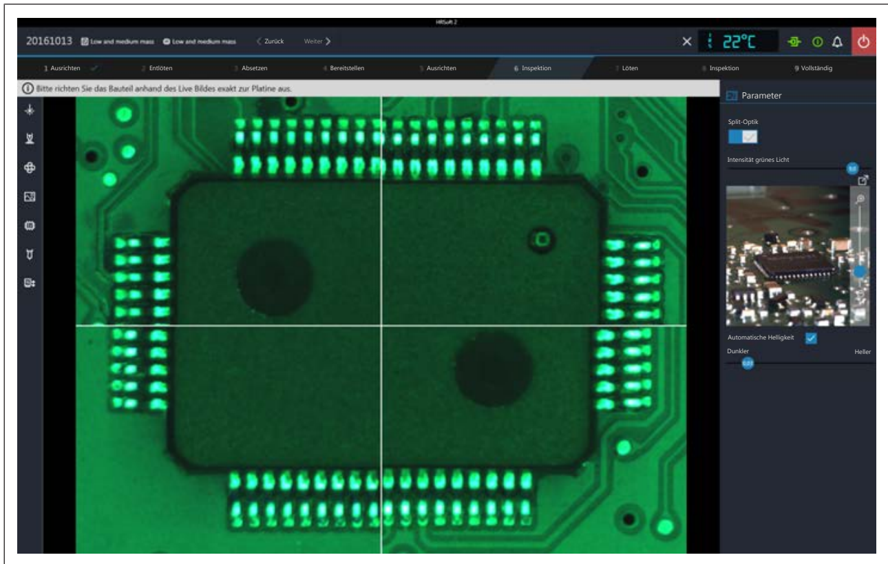
Abb. 43: Splitscreen-Ansicht mit gleichzeitiger Darstellung der vier Ecken eines großen Bauteils
