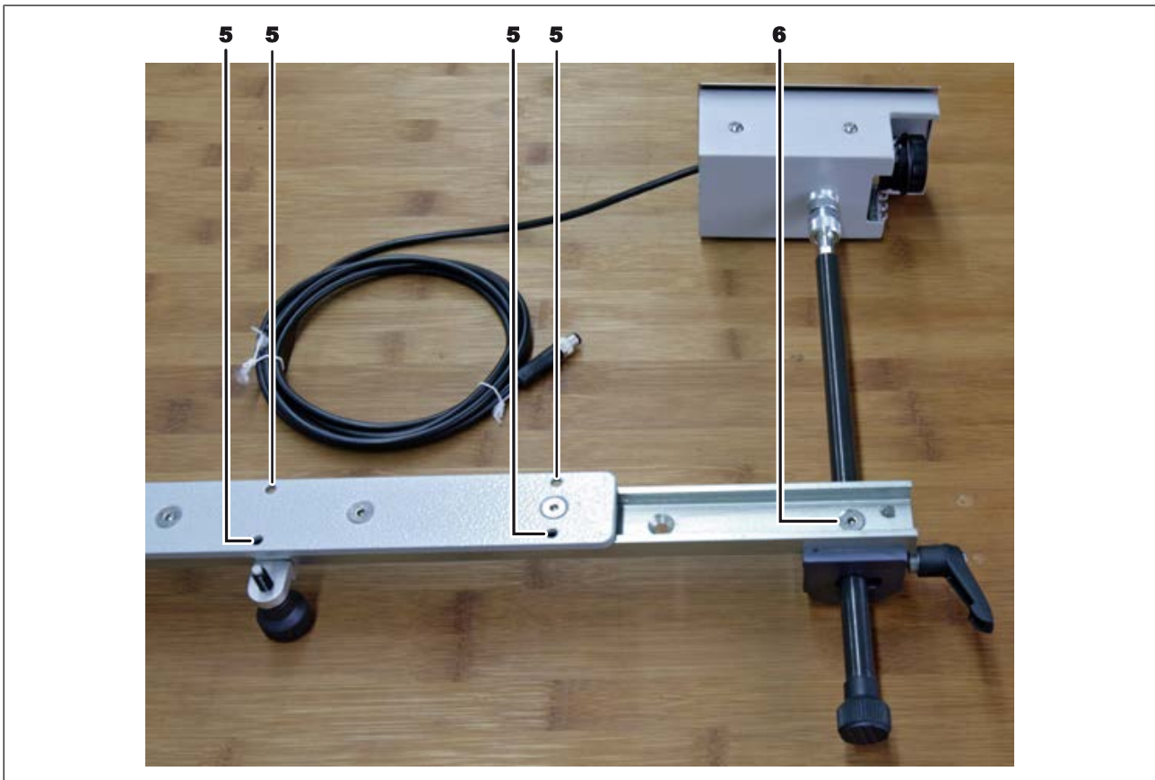
Abb. 7: RPC-Kamera zusammengebaut
