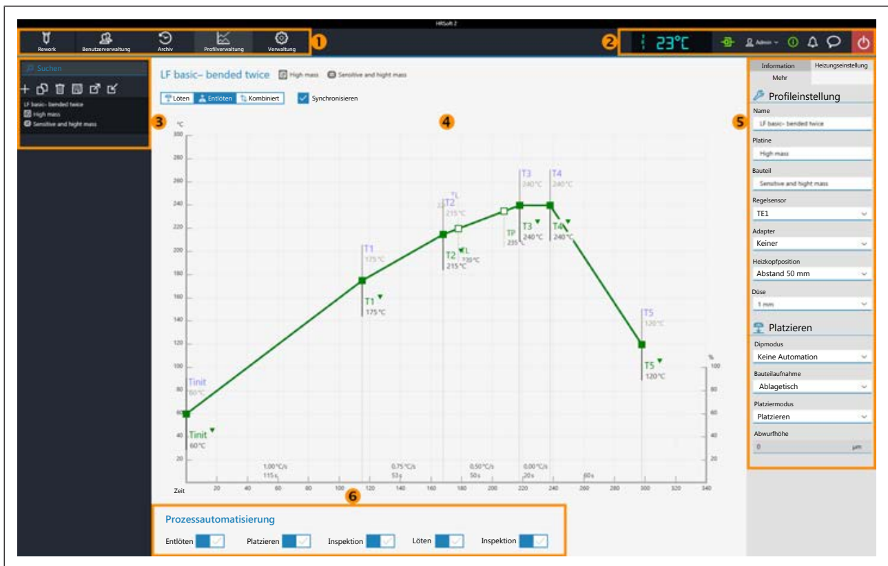
Abb. 28: Bereiche im Tabulator Profilverwaltung
