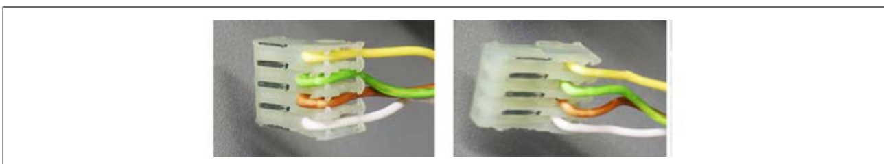
Abb. 19: Beispielabbildung. Links: Kabel in die Zugentlastung eingedrückt. Rechts: Kabel lose.
