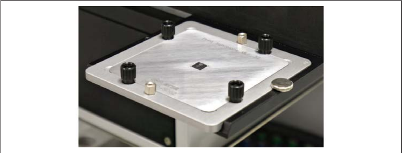
Abb. 39: Mit Lotpaste bestrichenes Bauteil in der Print-Schablone auf der Bauteilablage
