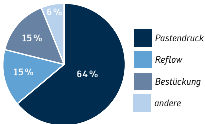
Fehlerverteilung im SMD-Prozess nach C. H. Mangin
